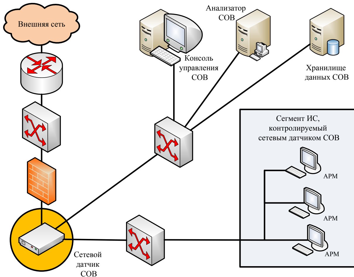
Рисунок 2.1 – Типовая схема применения в ИС СОВ уровня сети
